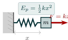
Figur 5.6: Komprimert fjær med kompresjon x . Fjærkraften F = kx skyver klossen vekk. Arbeidet W = \frac{1}{2}kx^2 er lagret som elastisk potensiell energi.
