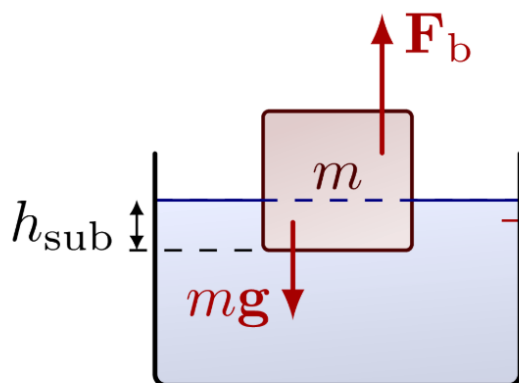
Figur 7.6: Oppdrift F_b , hvor oppdriftskraften beregnes ut fra volumet av væsken som fortrenses. Det fortrengte volumet er gitt som V_q = h_{\text{sub}} \cdot A , der h_{\text{sub}} er dybden av den nedsenkede delen av legemet, og A er arealet av bunnflaten.
